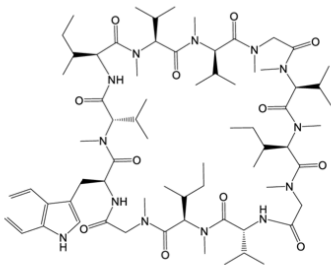
Omphalotin A (47)
